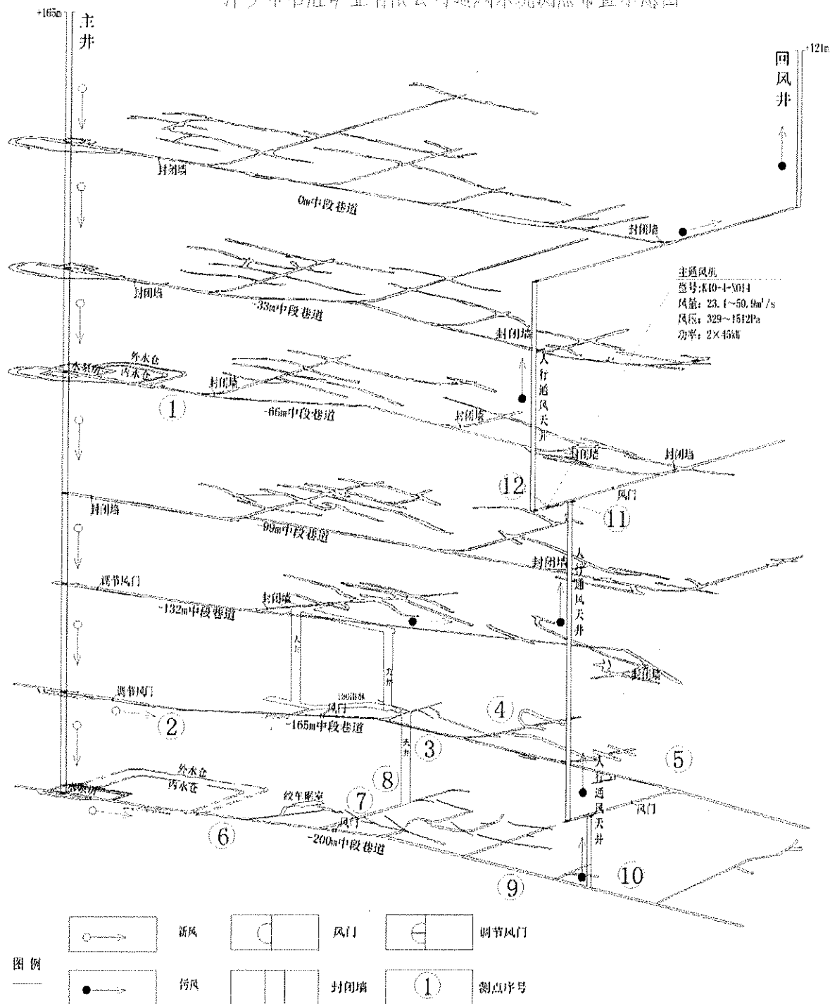
萍乡市名胜矿业有限公司通风系统测点布置示意图
